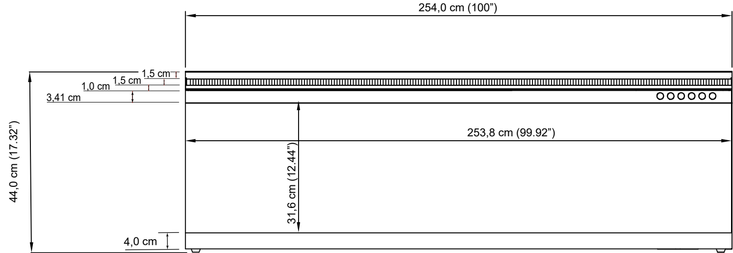
Bovenaanzicht
