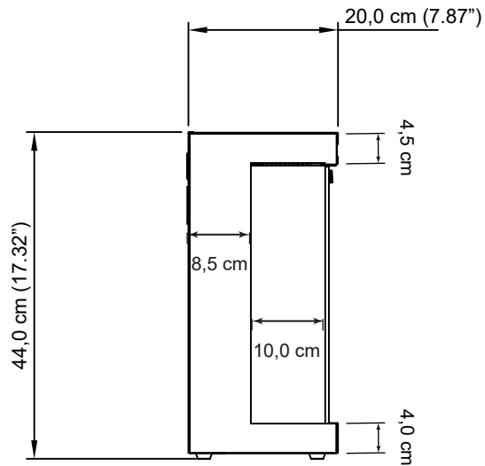
Zijaanzicht
