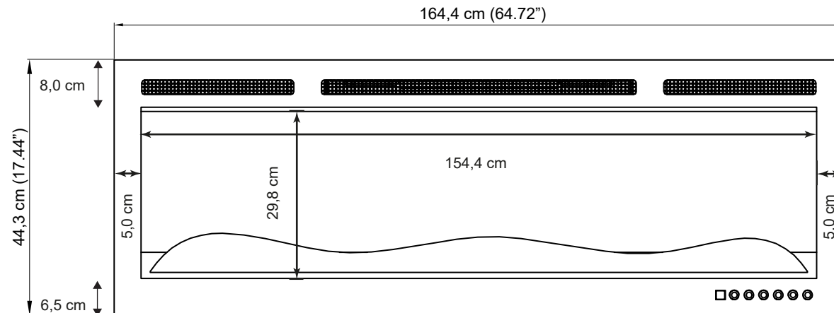
Vooraanzicht
