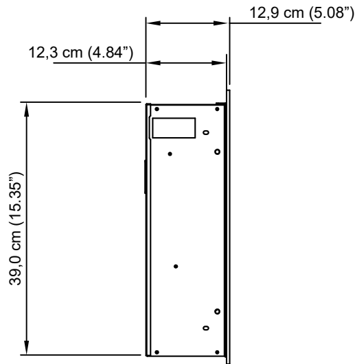
Zijaanzicht
