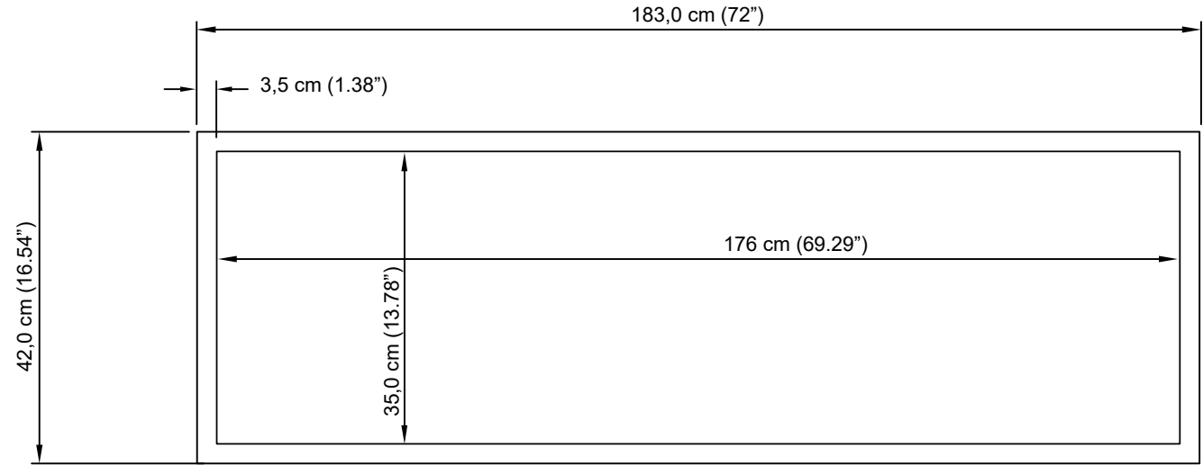
Bovenaanzicht
